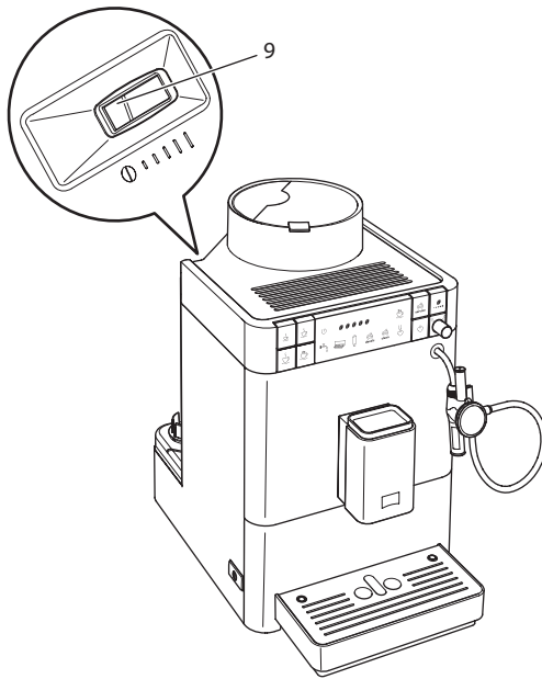
Fig. 13: Levier de réglage de la finesse de la mouture
