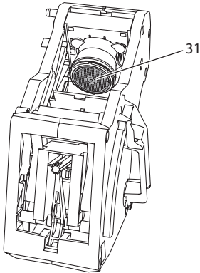
Kuva 15: Suodatusyksikön puhdistaminen
