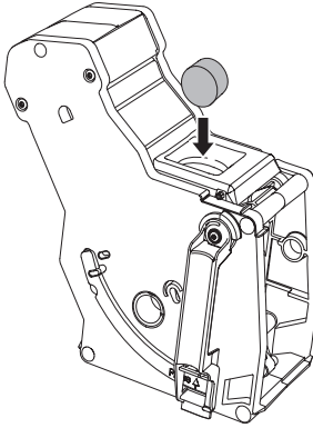
Resim 17: Temizleme tabletinin pişirme ünitesine yerleştirilmesi.
