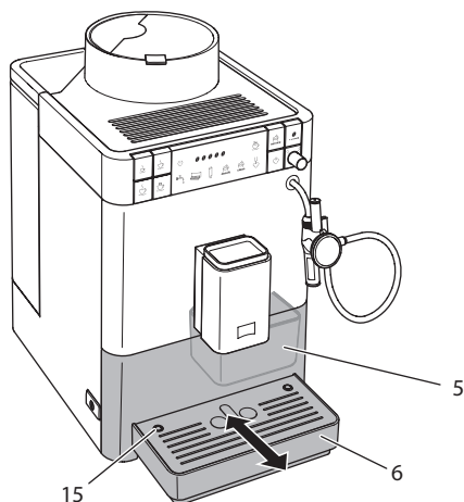
Pav. 11: Lašų surinktuvą ir kavos tirščių talpyklą ištuštinimas
