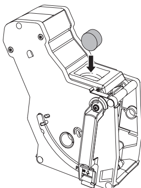
Bilde 17: Legg en rengjøringsstablett inn i kokegruppen.
