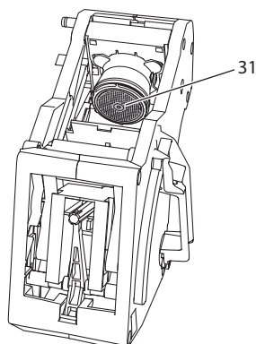
Fig. 15: Rengøring af brygheden
