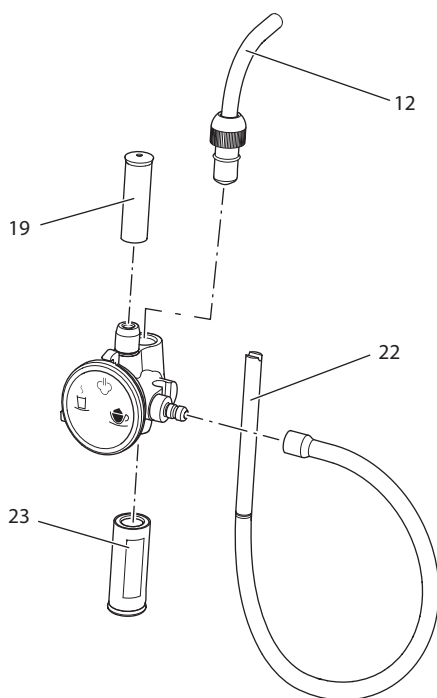
Fig. 16: Adskille cappuccinatoren
