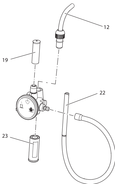
Fig. 16: Dezasamblarea cappuccinatorului
