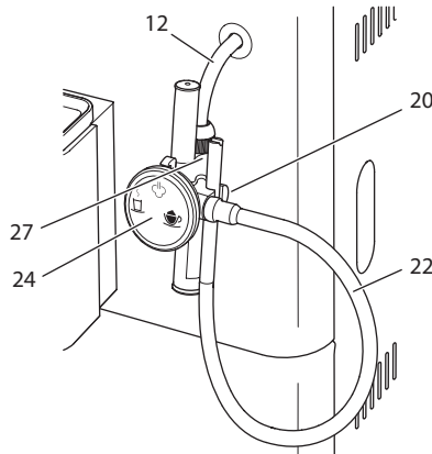
Resim 9: Cappuccinatore ünitesinin bağlanması
