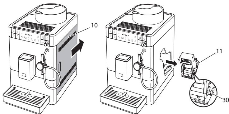
Fig. 14: Udtage brygheden
