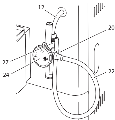
Kuva 9: Cappuccinatoren kytkeminen
