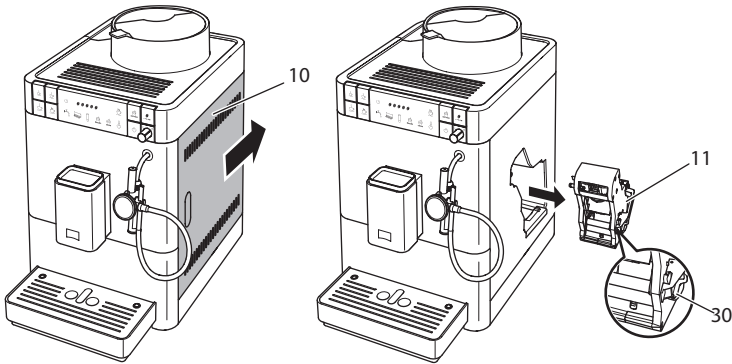
Fig. 14: Scoaterea unității de infuzare
