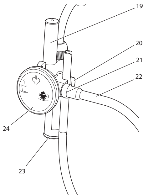
Pav. 4: Kapučinatorius
