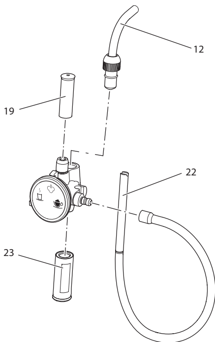
Pav. 16: Kapučinatoriaus išardymas
